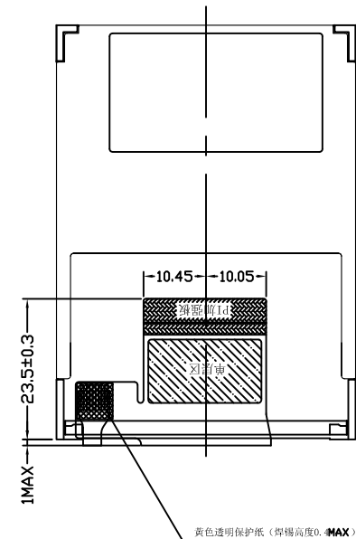
FPC折弯后示图 展开出货
